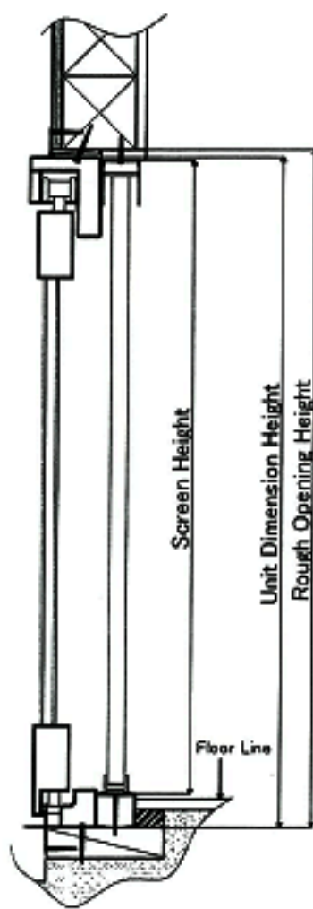
< A-A' Section >
