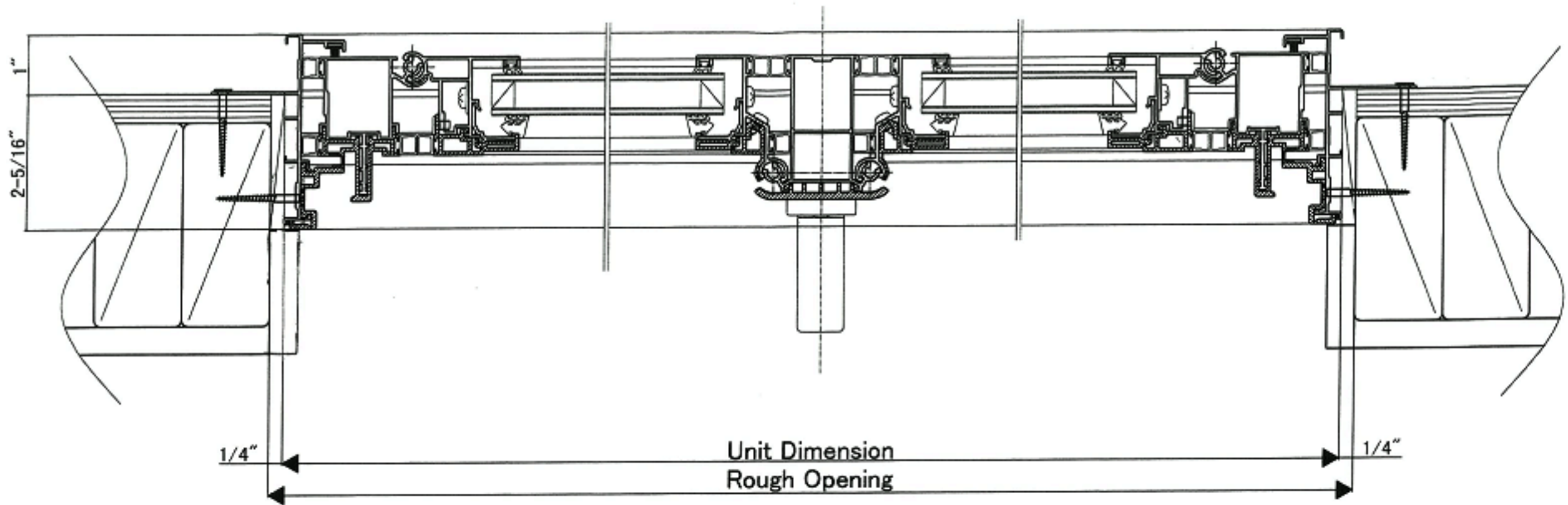
Bi-Fold Door 【Horizontal Drawing】
