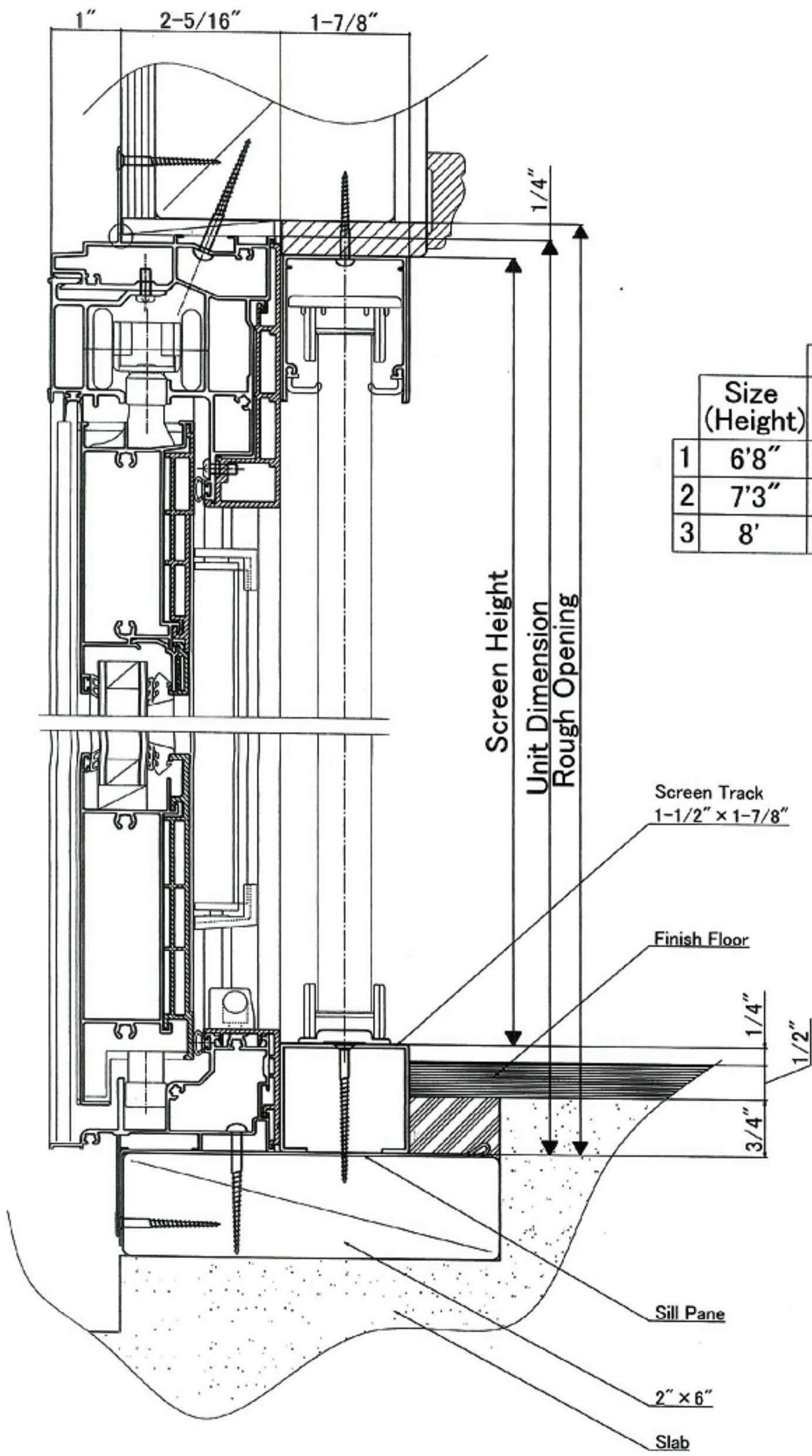
Bi-fold Door 【Vertical Drawing 1 】
