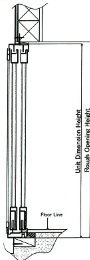
< A-A' Section >
