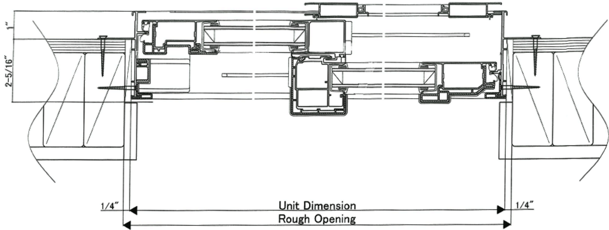
Double Sliding Door 【Horizontal Drawing】
