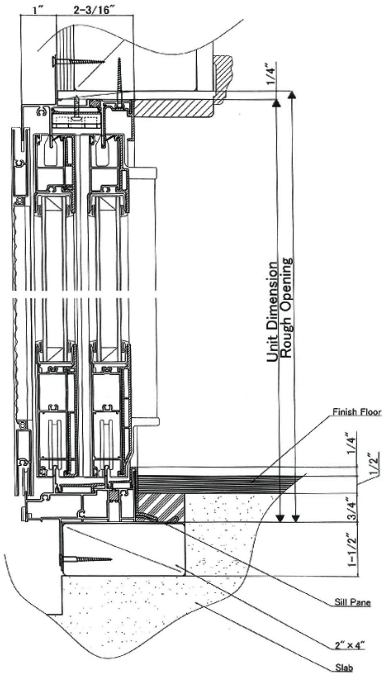
Double Sliding Door 【Vertical Drawing】
